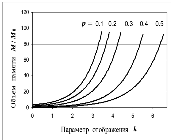
Рис.3 Рост объема памяти с ростом параметра отображения k ( p=0.1 \div 0.5 ).
